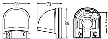
※当社Gタイプコネクタ(16・22・28)が取り付けられます。
