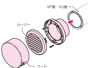
防虫ネット付 (樹脂8メッシュ)
