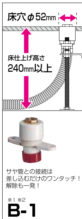
たて型水栓ジョイント本体
