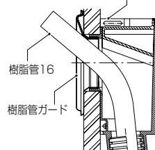
水栓ジョイントボックス
