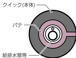
立断面図
