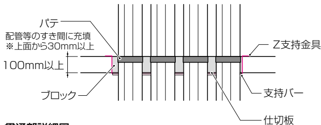
貫通部詳細図
