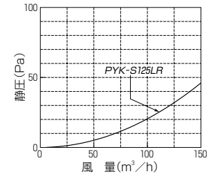
圧力損失特性(排気)
