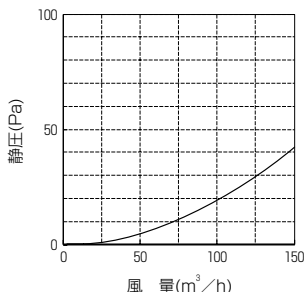
圧力損失特性
