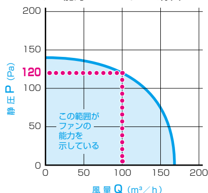
ファン能力をあらわすP-Q線図
