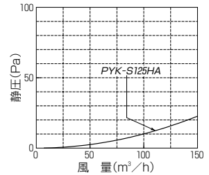
圧力損失特性(排気)
