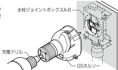
■ボックス探知工法に
