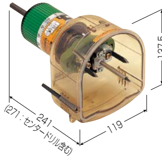
■ボックス探知工法に
