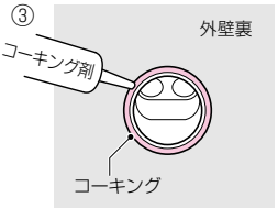
コーキング
