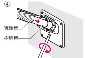
ねじ穴(φ4.5mm)
