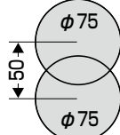
だるま穴
